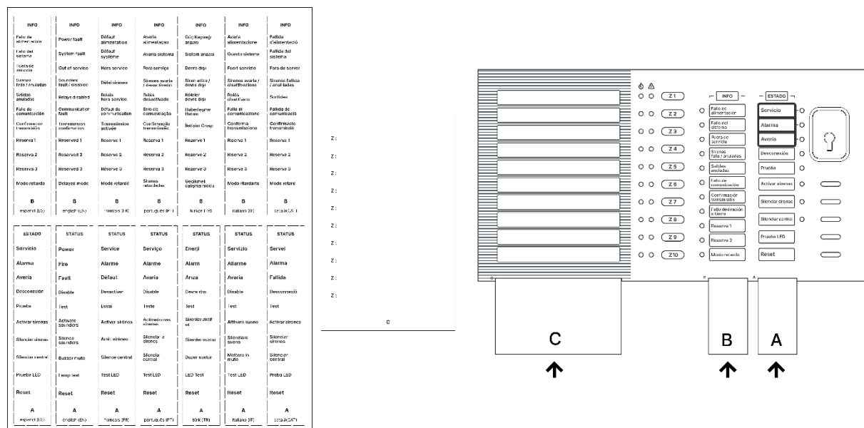
Fig. 9 Personalización de idioma y texto de zonas en Central CCE-200
