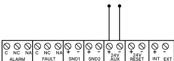
Fig. 23 Conexión Salida 24V auxiliar
