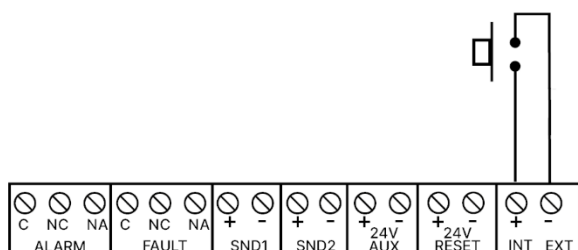
Fig. 22 Conexión Entrada auxiliar
