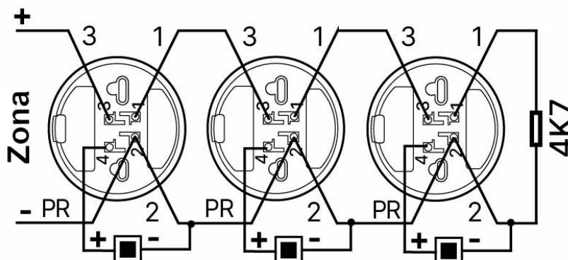
Fig. 19 Conexión de detectores con piloto indicador de acción
