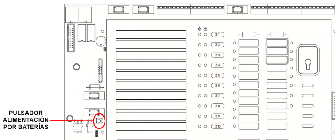
Fig. 37 Pulsador alimentación por baterías
