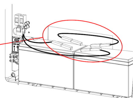
Fig. 15 Conexión de las baterías
