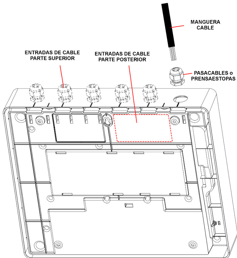
Fig. 7 Zonas previstas para entrada de cable en parte trasera y superior.
