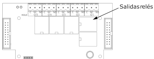
Fig. 36 Tarjeta de expansión de 5 salidas de relé TRE-200
