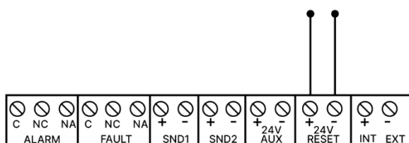
Fig. 24 Conexión Salida 24V rearmable
