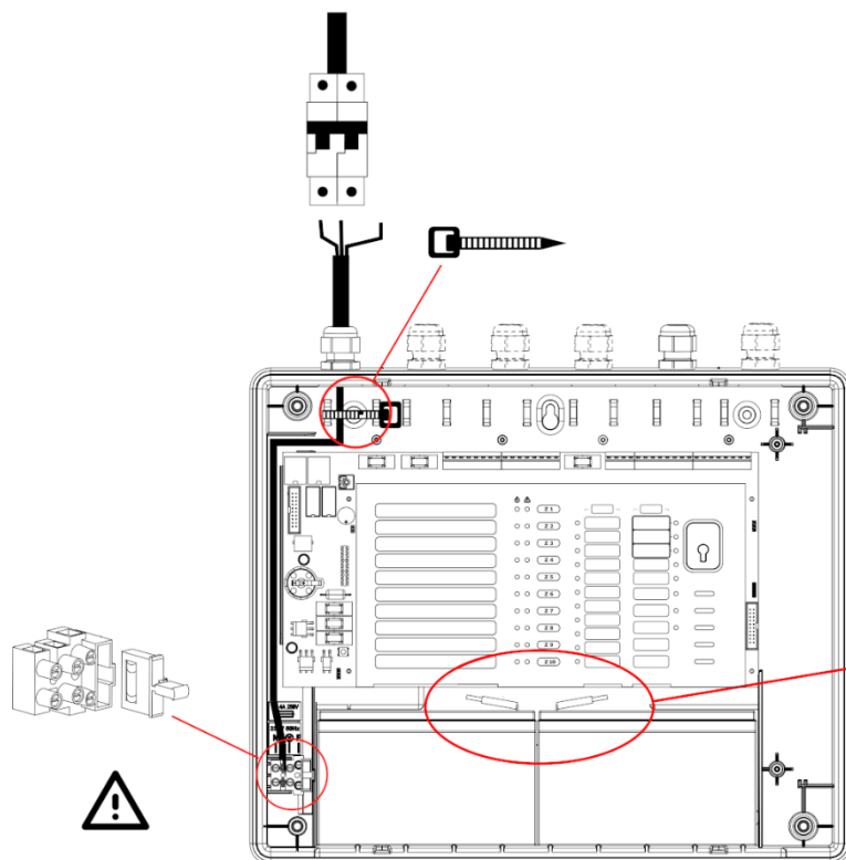
Fig. 13 Alimentación a 230 VAC
